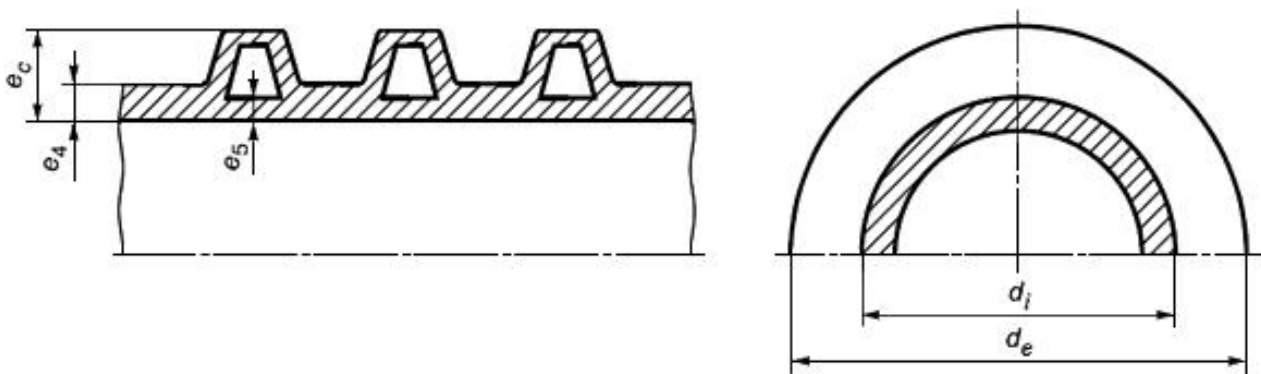
е) Тип В (с кольцевым полым профилем)
